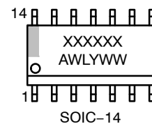
SOIC-14
